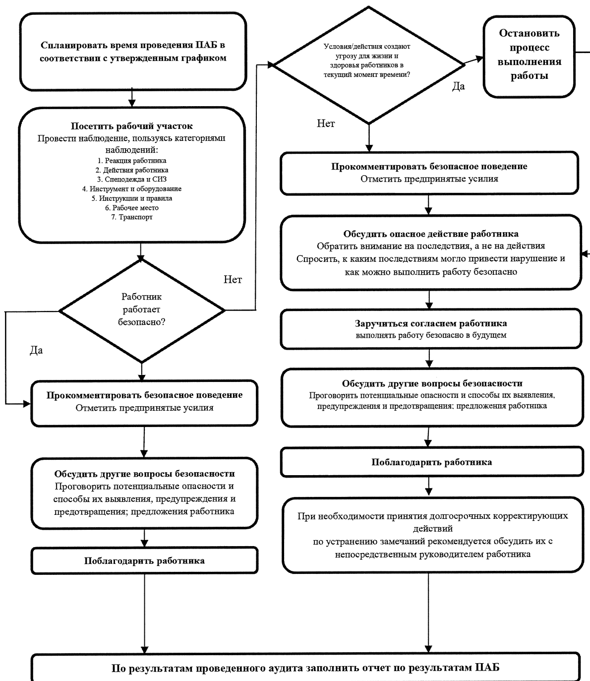
Рисунок 1 – Блок-схема порядка проведения ПАБ
